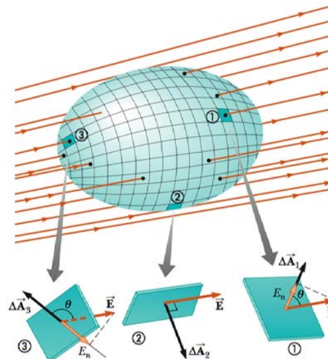
Figura 2.3: Fluxo elétrico através da superfície A . O fluxo é positivo, zero e negativo nos pontos 1, 2 e 3 respectivamente, de acordo com o ângulo \theta . (Serway)
